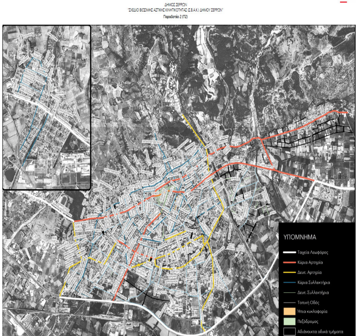
Σχήμα 4.2: Λειτουργική ιεράρχηση οδικού δικτύου
